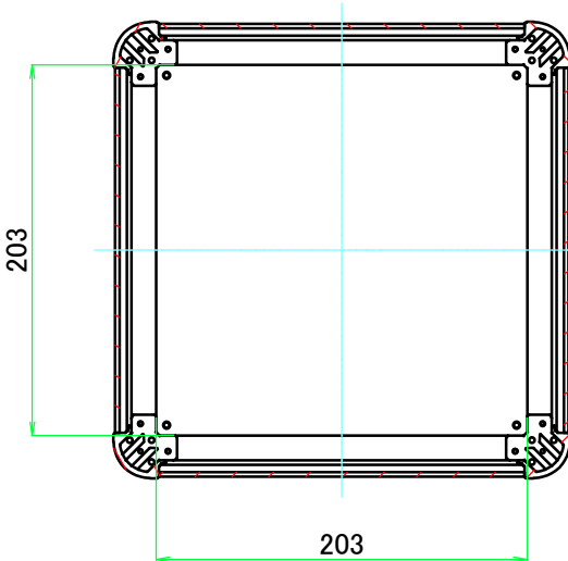
C-C ( 1 : 4.5 )
