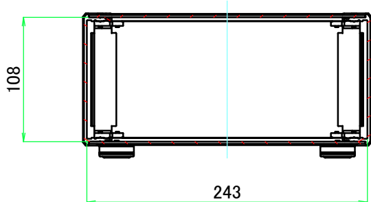
A-A ( 1 : 4.5 )
